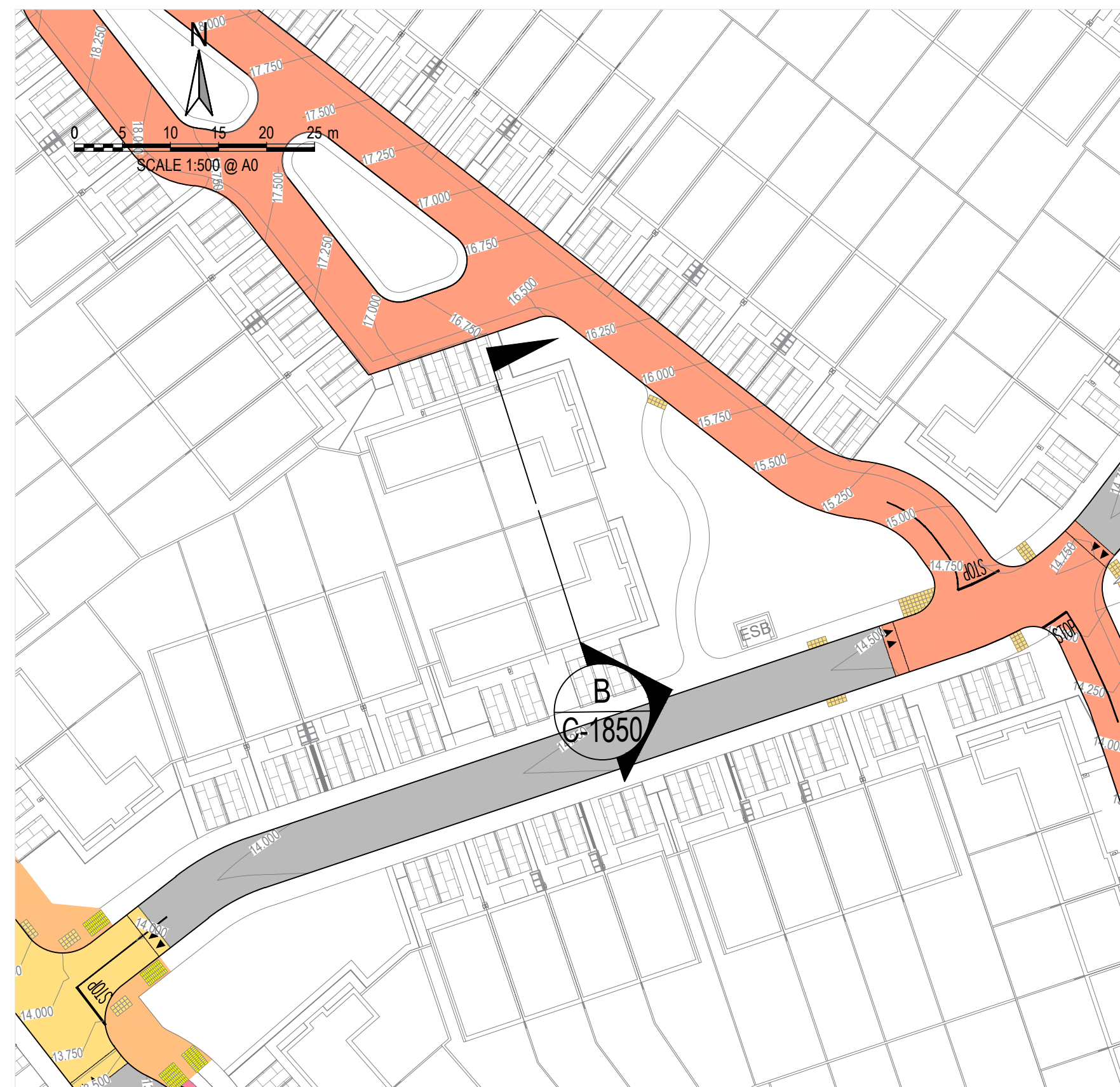
KEYPLAN - SECTION B SCALE: 1:500
