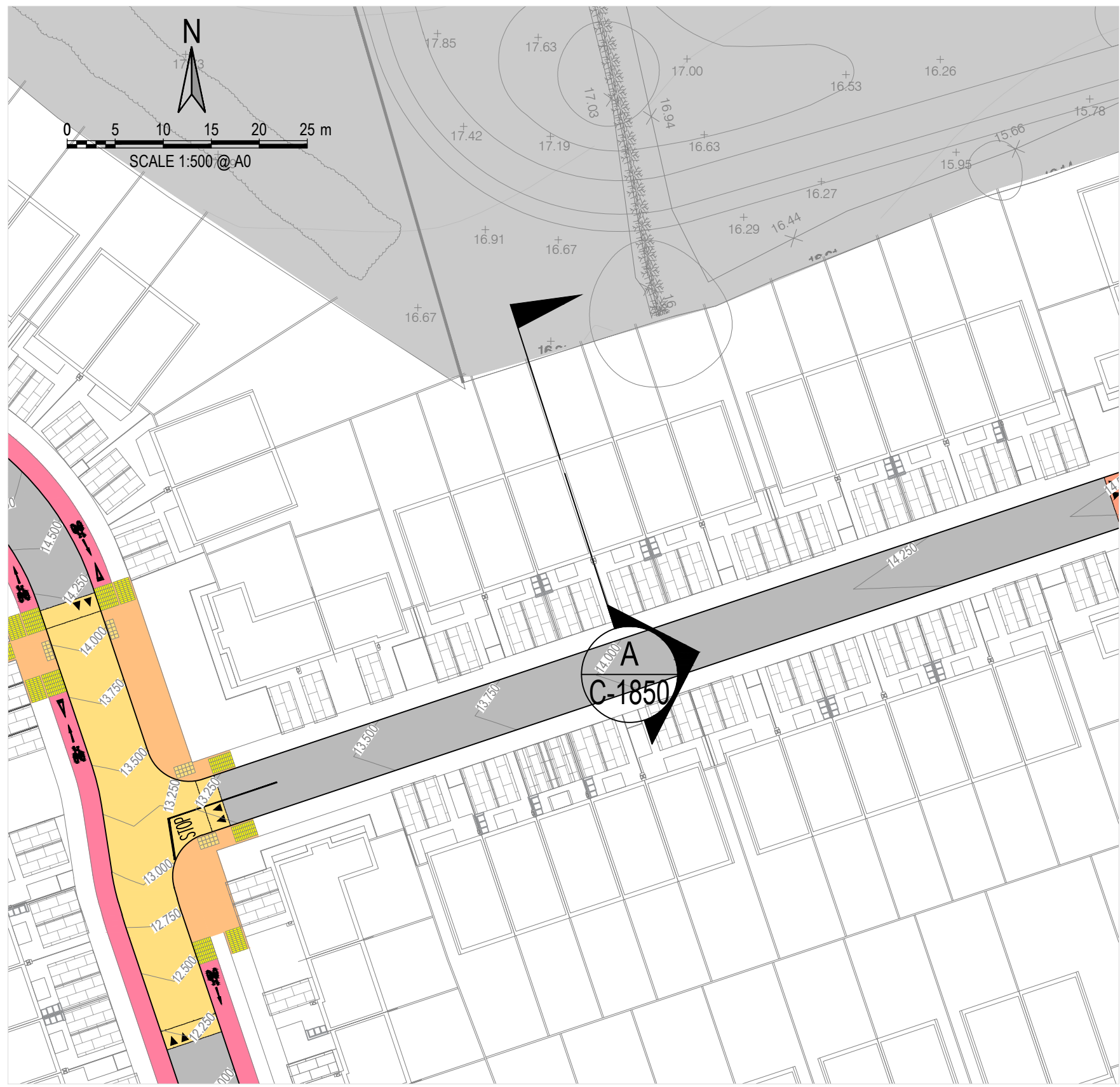
KEYPLAN - SECTION A SCALE: 1:500
