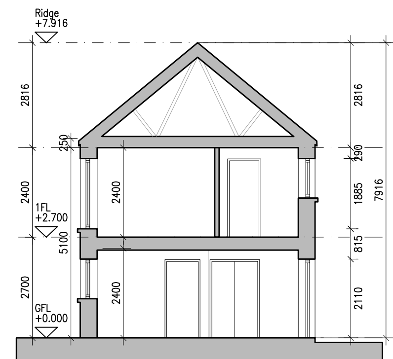
14 Type F2 - Section AA 207 1:100@A1 3 BED HOUSE
