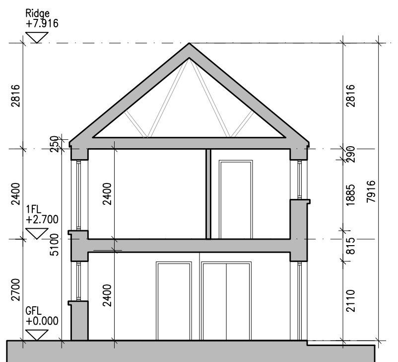
07 Type F1 - Section AA 207 1:100@A1 3 BED HOUSE
