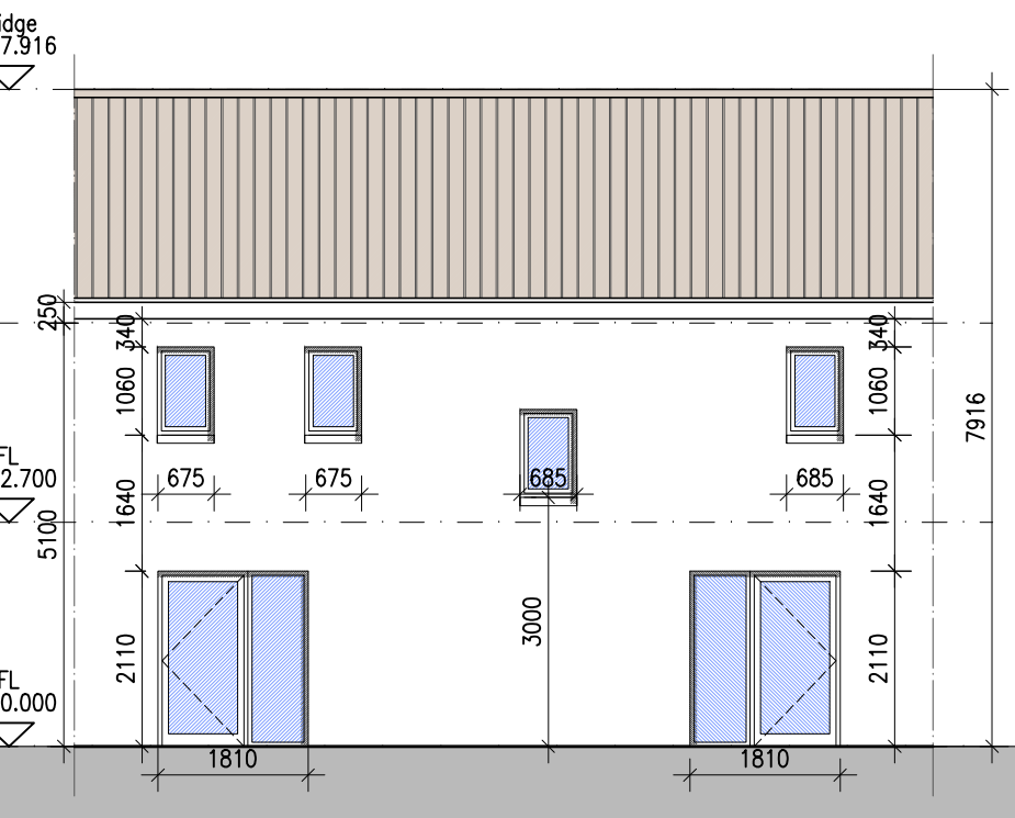
06 Type F1 - Rear Elevation 207 1:100@A1 3 BED HOUSE
