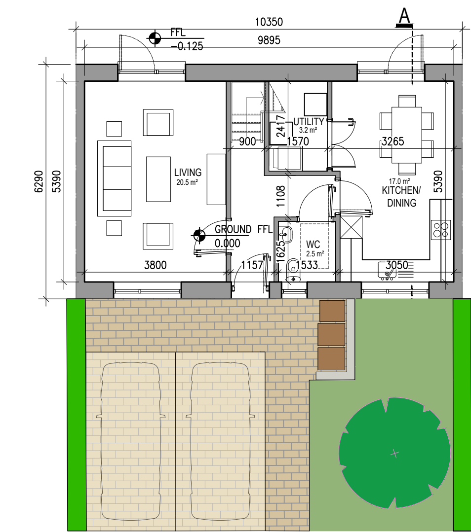
01 Type F1 - Ground Floor Plan 207 1:100@A1 3 BED HOUSE
